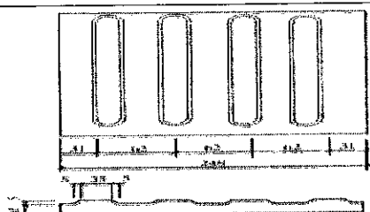
图2 行进盲道
