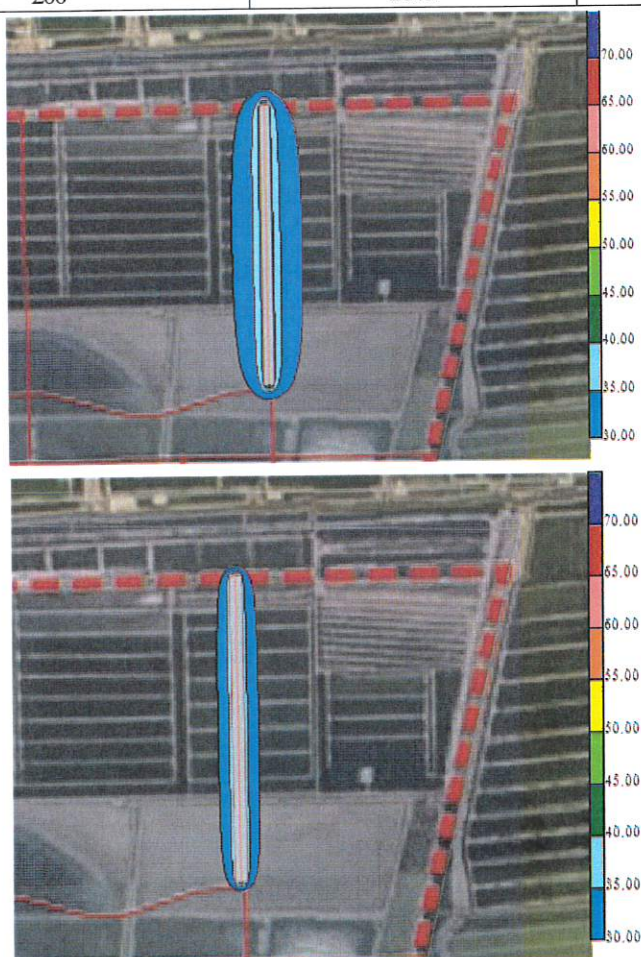
图 13 运营期交通噪声预测等值线图（昼、夜）
