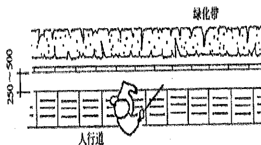
图2 行进盲道
