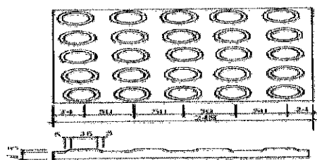
图3 提示盲道
