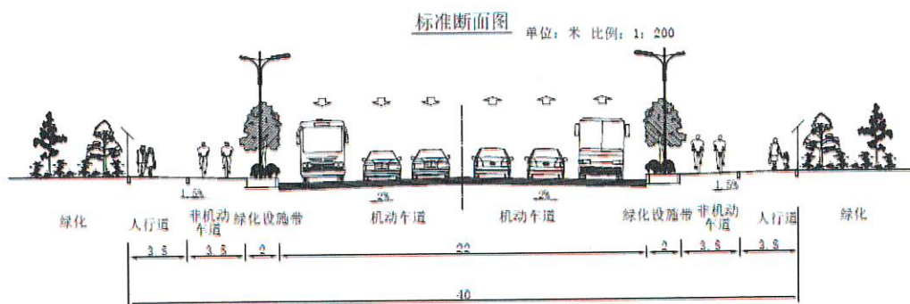
图1 标准横断面
